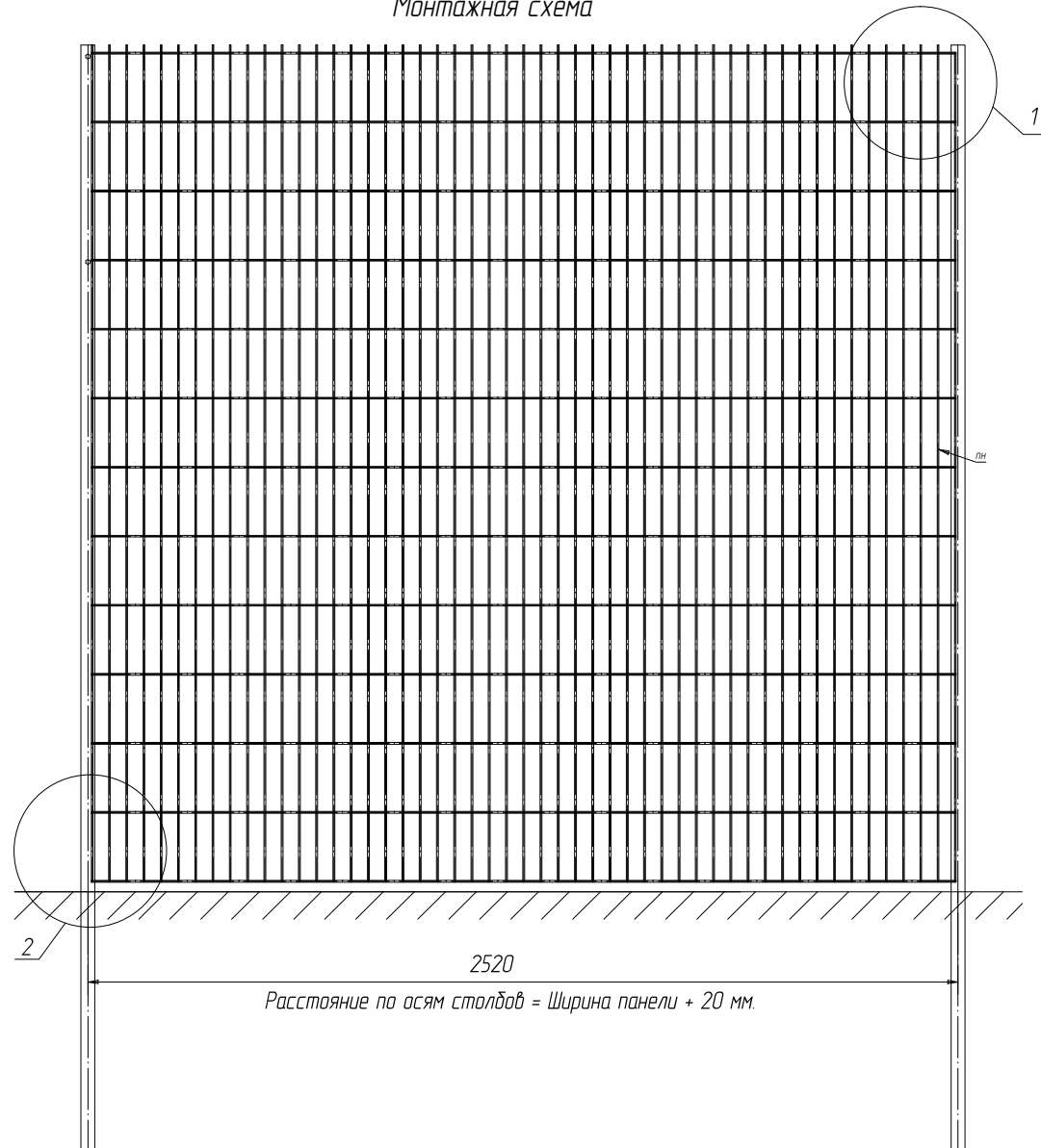
Монтажная схема
