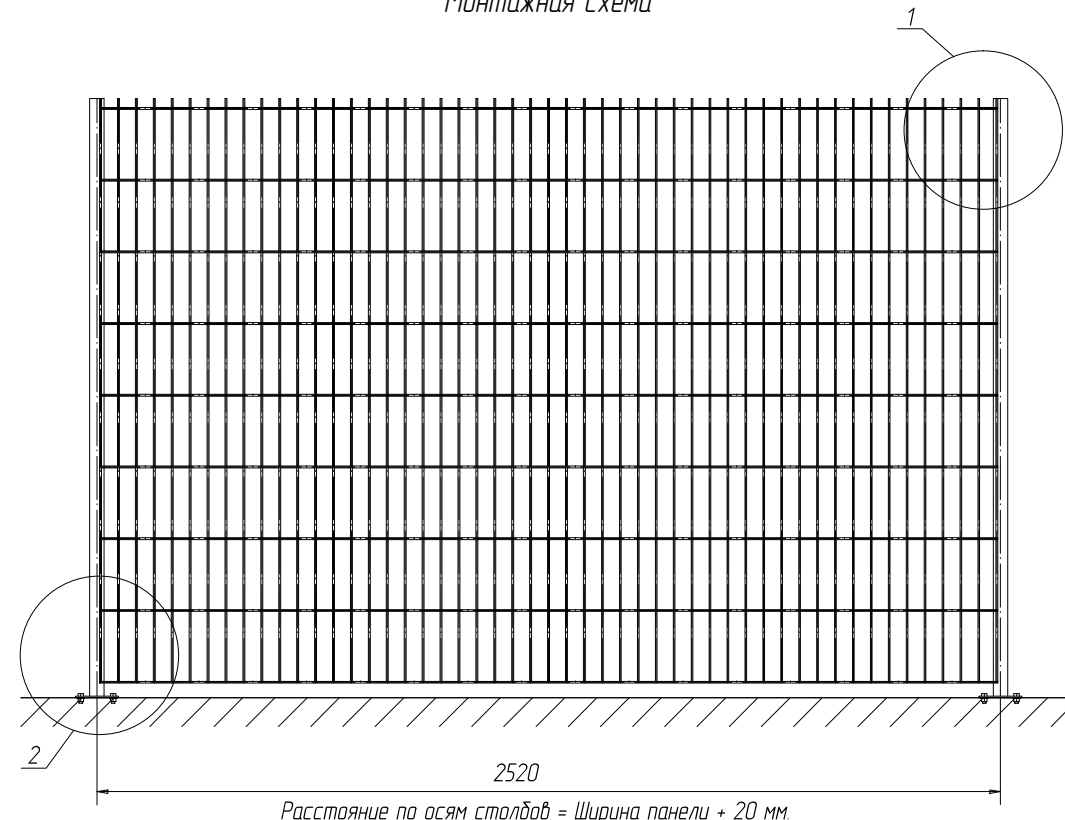
Монтажная схема
