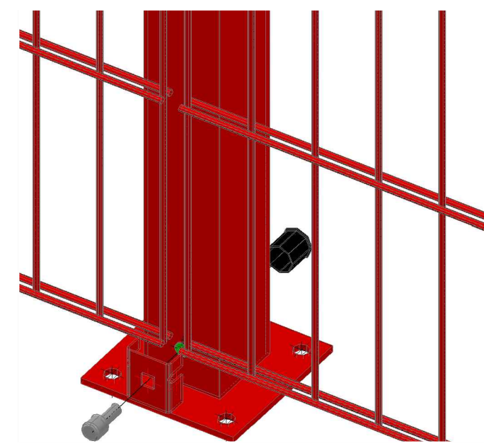
Узел - 2
