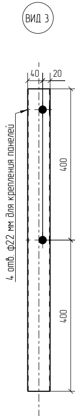
Столб угловой
