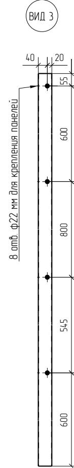
Столб угловой
