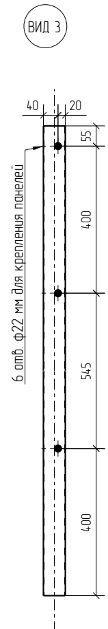
Столб угловой
