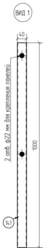
Столб промежуточный
