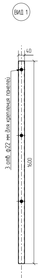
Столб промежуточный
