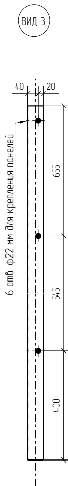
Столб угловой
