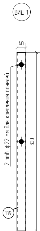
Столб промежуточный
