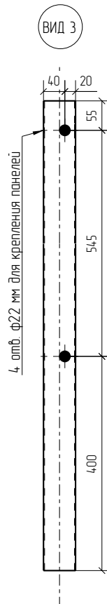
Столб угловой
