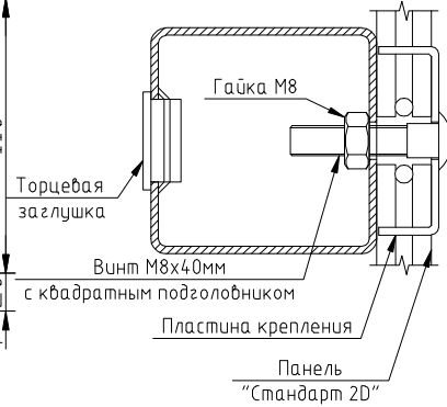
Схема крепежа (тип 3φ) М 10:1
