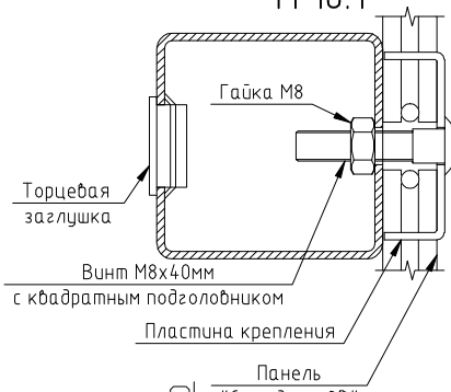
Схема крепежа (тип 3д) М 10:1
