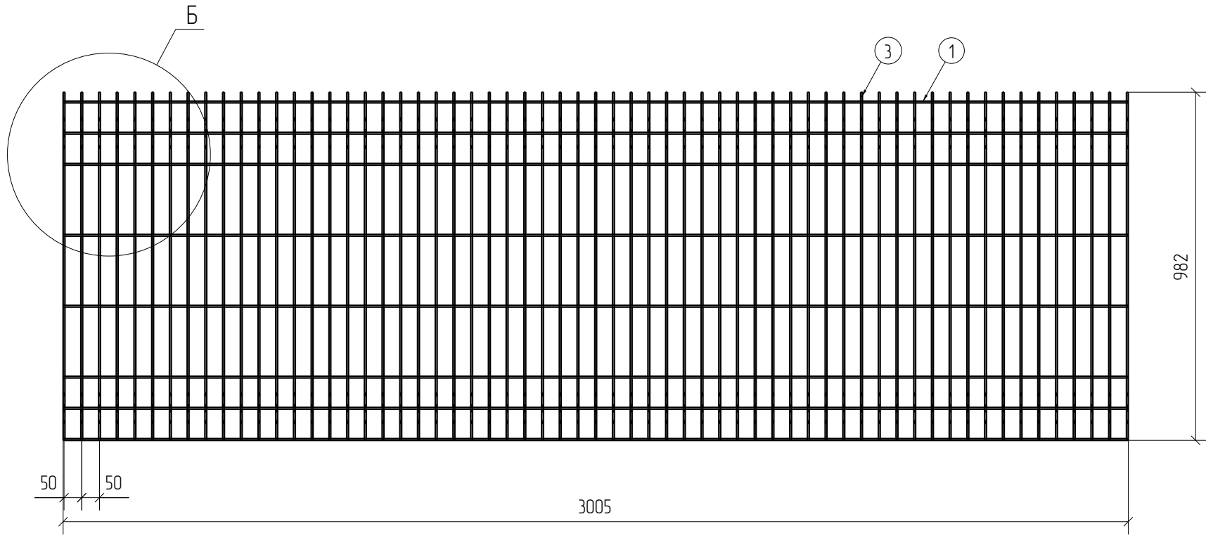
ПН.ЗД.5.50x200.3000x982.ГЦ
